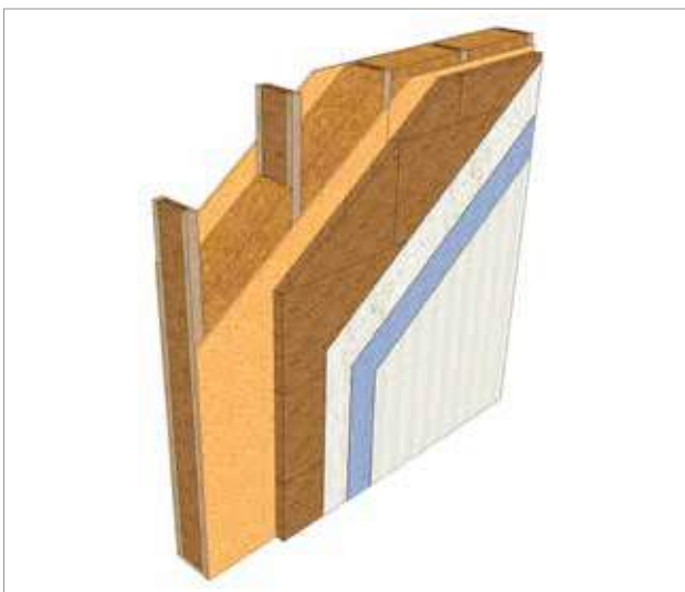
Ossature bois avec contreventement extérieur
