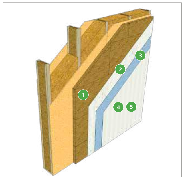
Ossature bois avec contreventement extérieur
