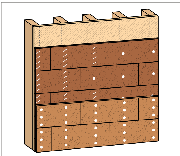
Sur ossature bois avec contreventement extérieur
