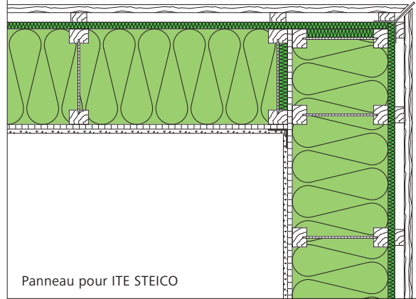
W2 Angle de mur extérieur avec STEICOjoist
