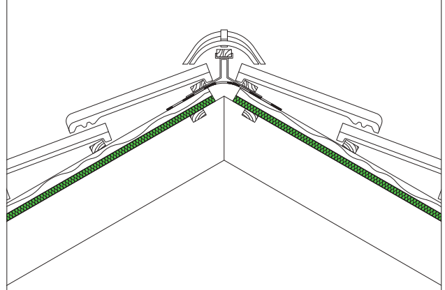
D4 Faîtage ventilé
