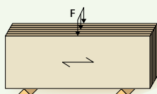
A f_{m,0,edge} et E_{0,edge} À chant, parallèle au fil du bois ♦
