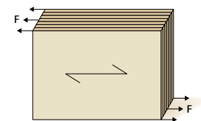
J f_{v,0,edge} et G_{0,edge} À chant, parallèle au fil du bois ♦
