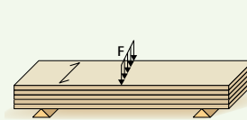
D f_{m,90,flat} et E_{90,flat} À plat, perp. au fil du bois ♦♦
