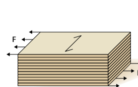
M f_{v,90,flat} et G_{90,flat} À plat, perp. au fil du bois ♦♦
